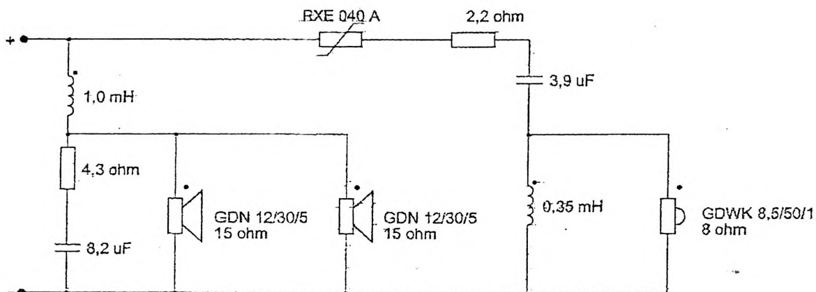
SCHEMAT ZWROTNICY ELEKTRYCZNEJ
