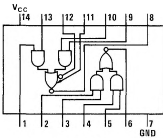
DM74H50
