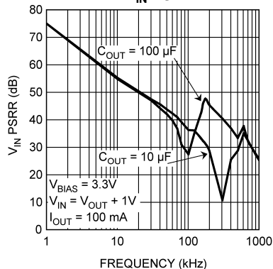
V_{IN} PSRR
