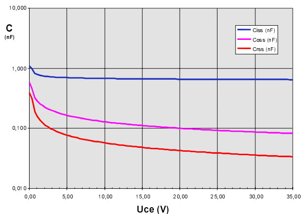
Typ. capacitances
