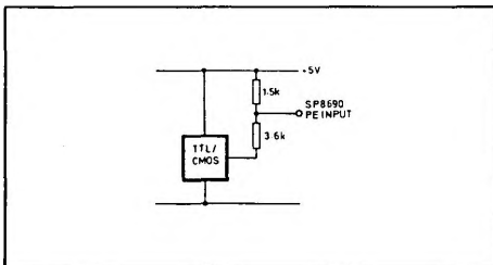
Fig.3 TTL/CMOS interface
