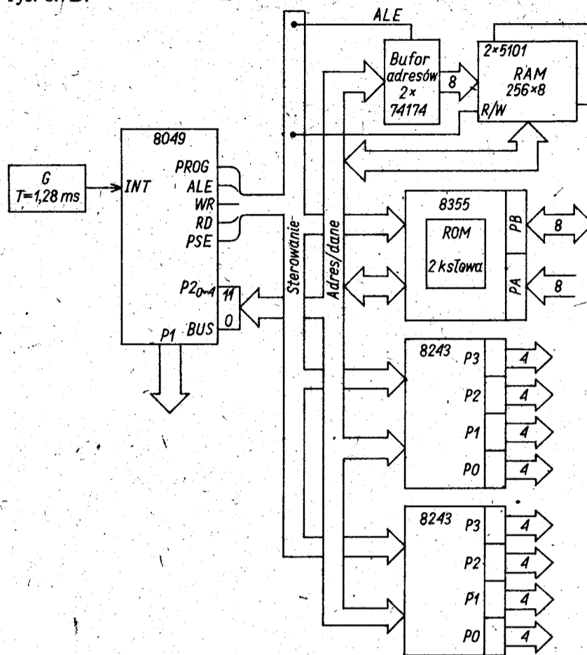
•8.7D• Uproszczony schemat mikrokomputera z magnetowidu VR 2020
