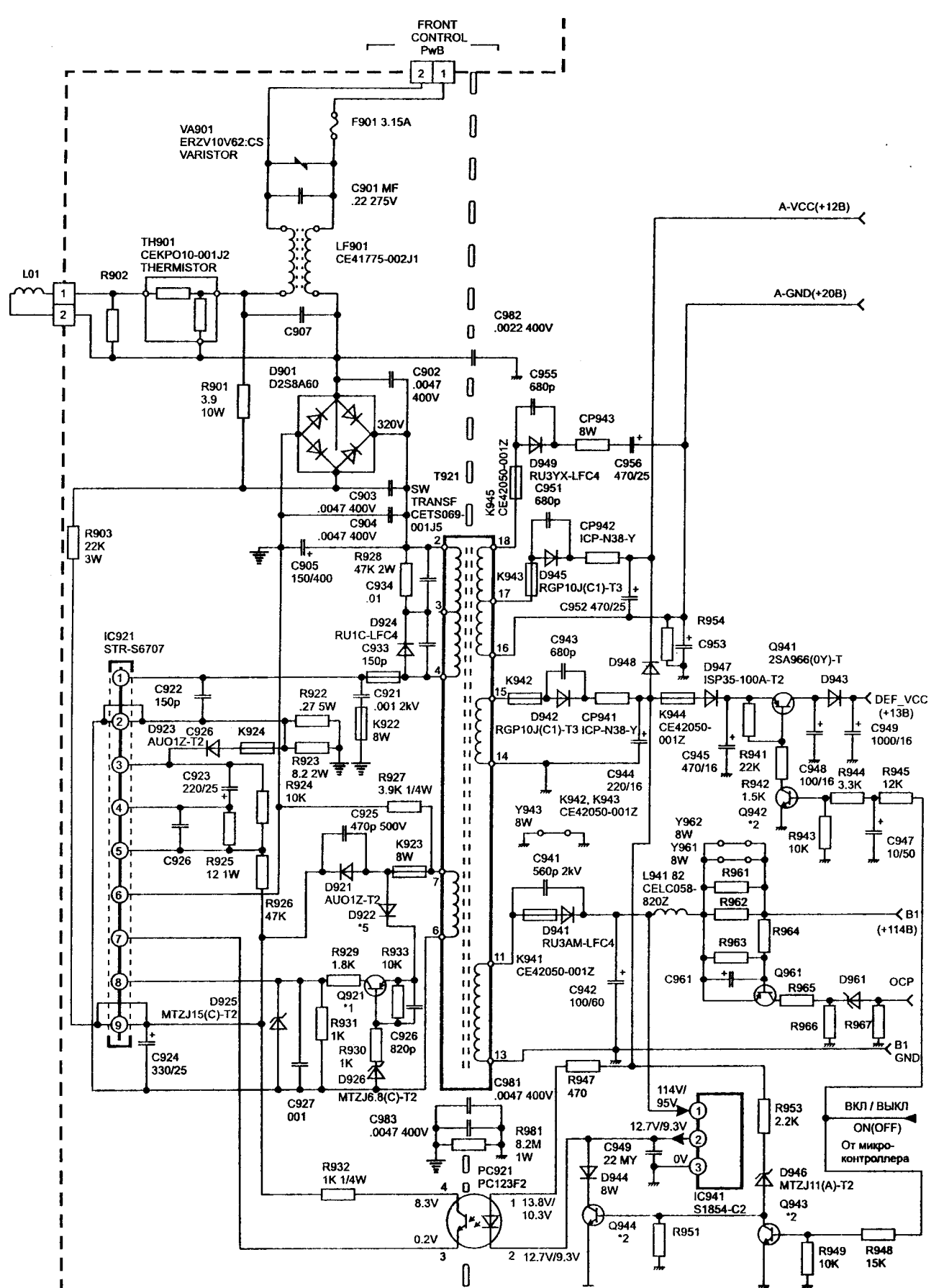
Принципиальная схема
